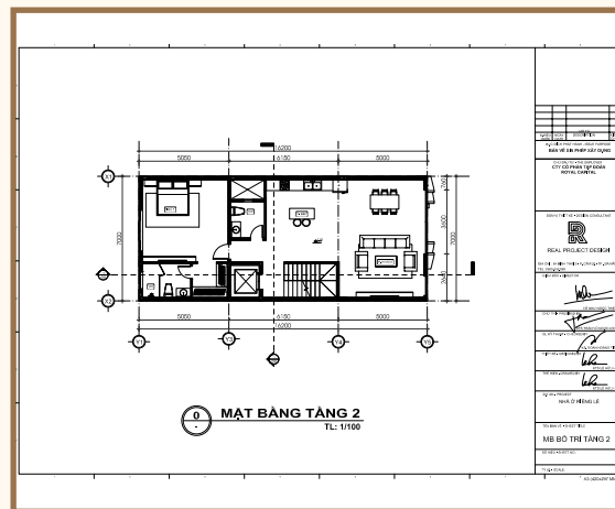
Mặt bằng T2
