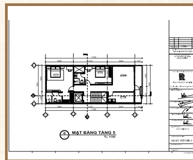
Mặt bằng T5
